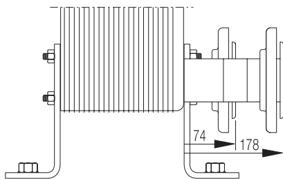
ANSI 300, Ø 3"
